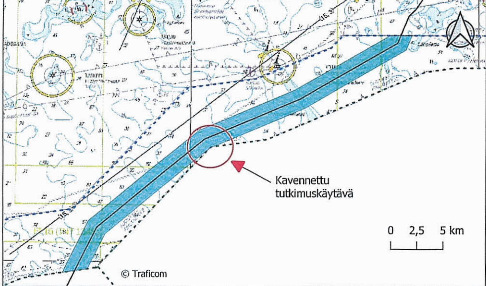
Kuva 3. Eastern Light -merikaapelin reitti ja tutkimuskäytävä Suomen talousvyöhykkeellä.
