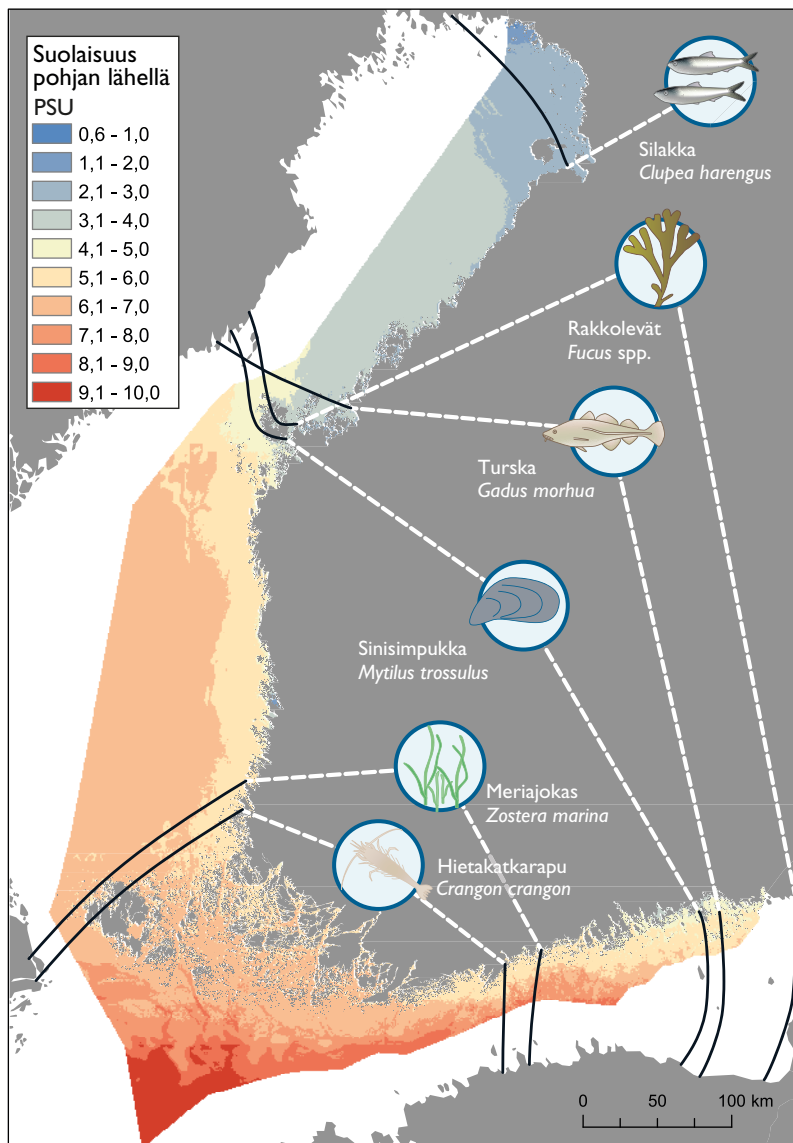
Kuva 1. Pohjan läheisen veden suolapi- toisuus ja eräiden avainlajien levinnei- syysrajat (Suomen ympäristökeskus, HELCOM).
